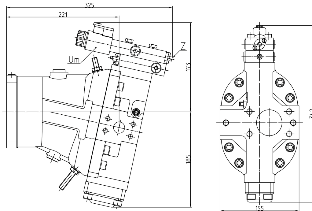
Рис. 60 – Габаритные и присоединительные размеры насосов 313.3(4).55
