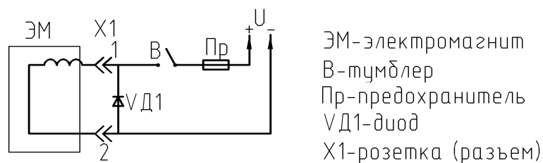
Рис. 43 – Схема подключения
