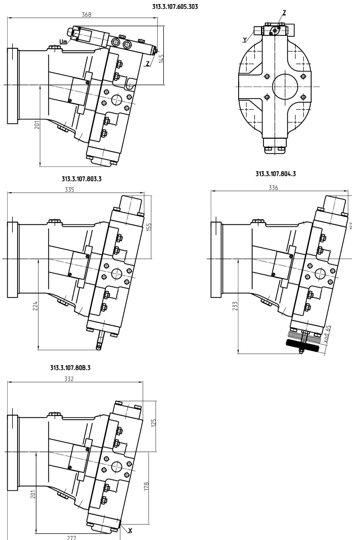
Рис. 71 – Габаритные и присоединительные размеры насосов 313.3(4).107
