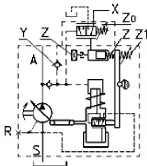
Рис. 19 – Гидравлическая схема насосов с регулятором постоянной мощности, позитивным управлением, ограничением предела верхнего реагирования и клапаном отсечки в серволинии.
