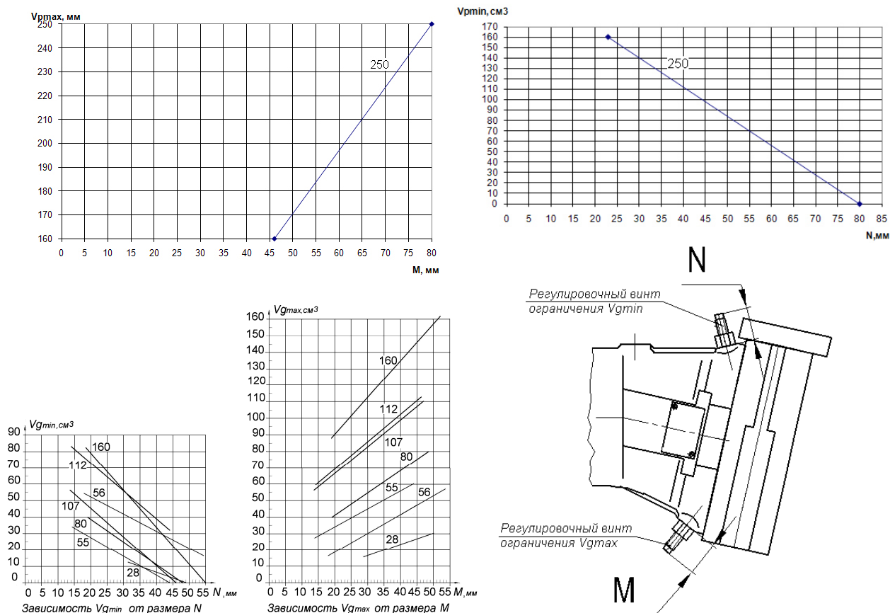
Рис. 4 – Ограничение максимального и минимального рабочего объема
