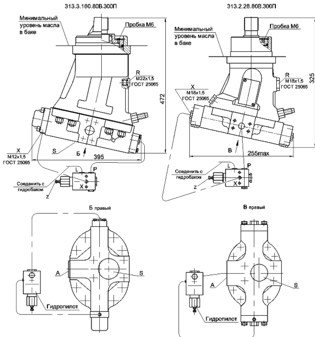
Рис. 41 – Схема соединения насосов с регулятором постоянного давления с дистанционным гидропилотом.
