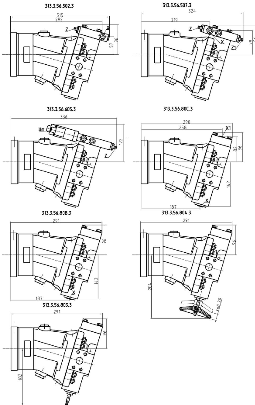
Рис. 62 – Габаритные и присоединительные размеры насосов 313.3(4).56
