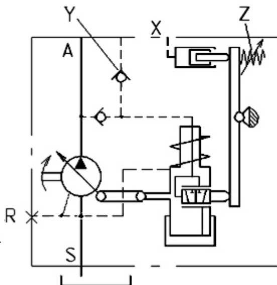
Рис. 26 – Гидравлическая схема насосов с регулятором постоянной мощности, гидравлическим позитивным управлением.
