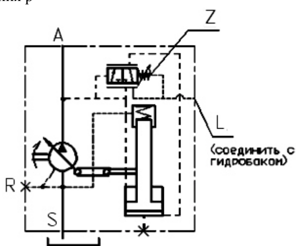
Рис. 16 – Гидравлическая схема насосов с регулятором постоянного давления с рабочим давлением 28 \text{см}^3 .
